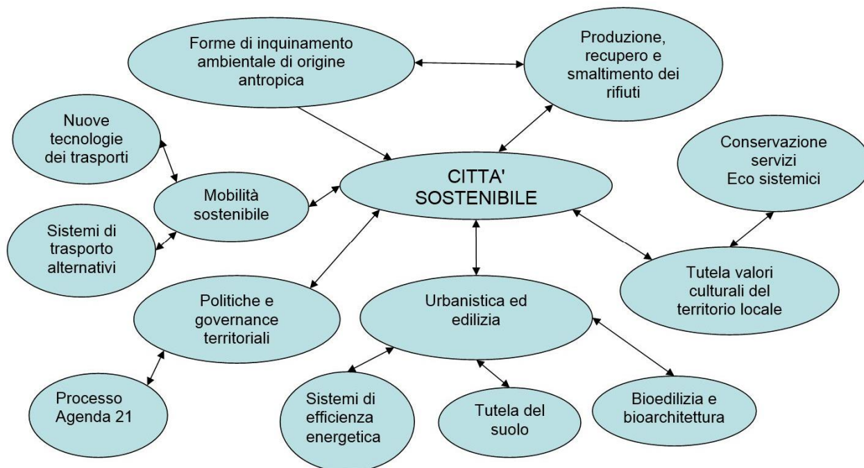
Mappa concettuale
