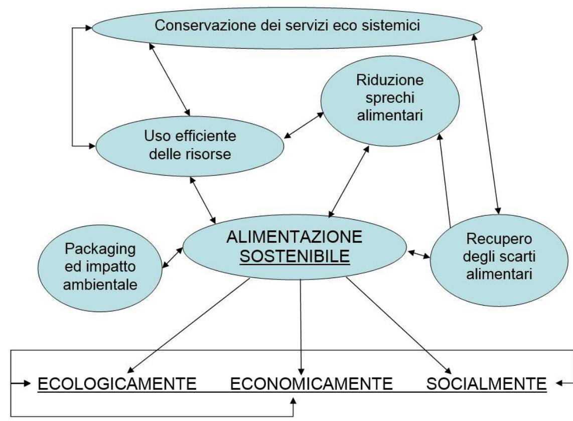
Mappa concettuale
