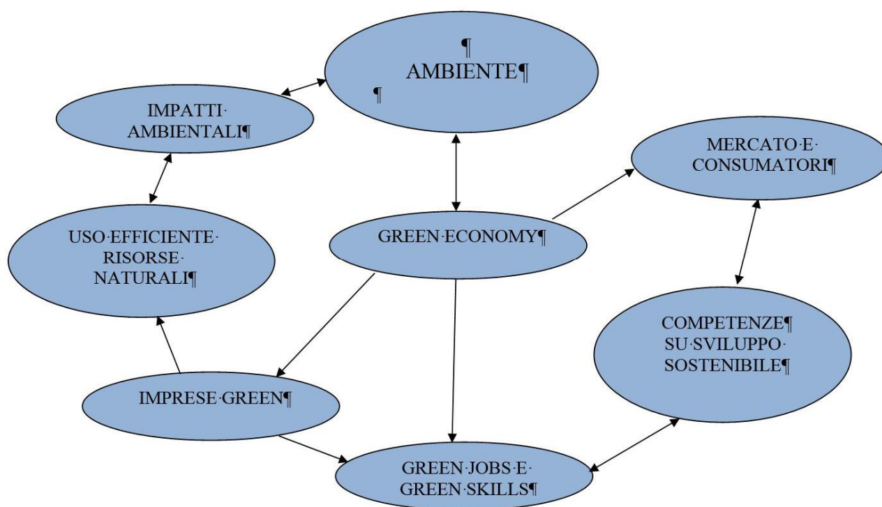
Mappa concettuale
