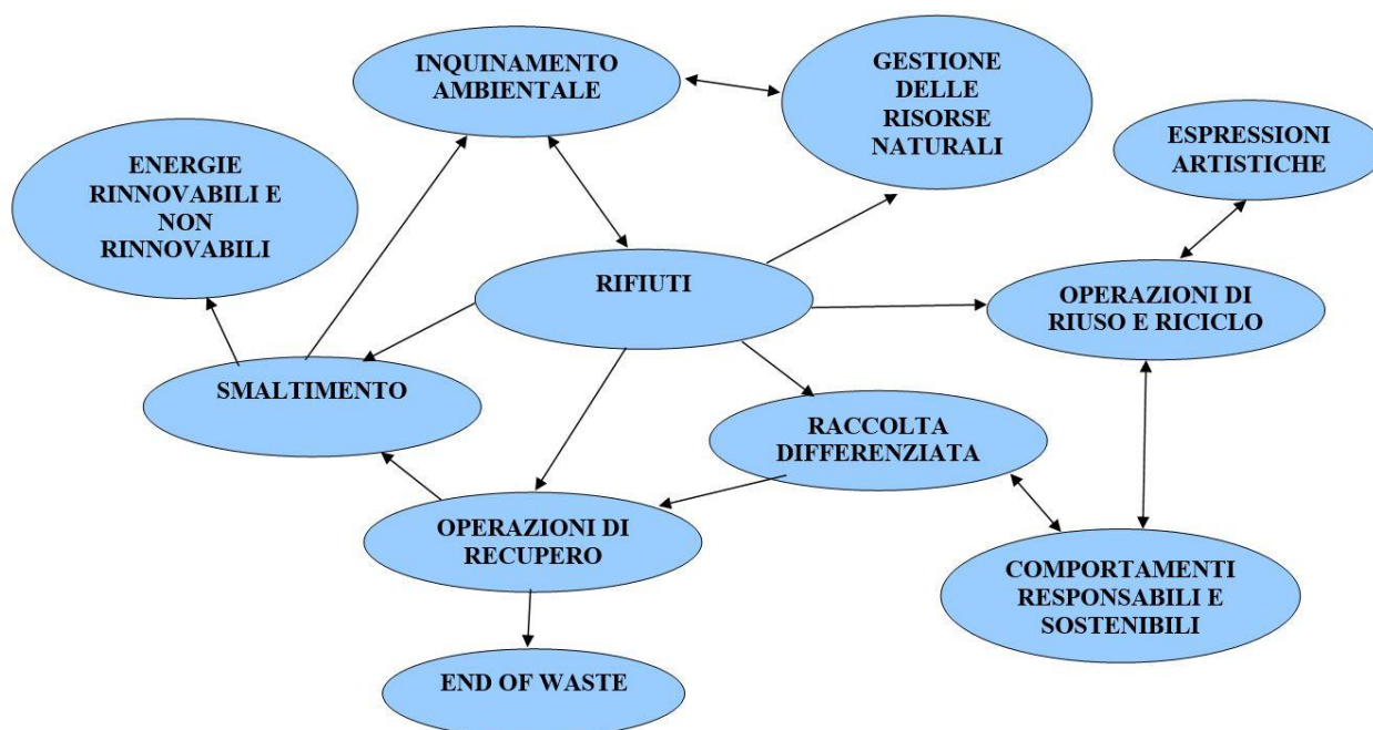
Mappa concettuale
